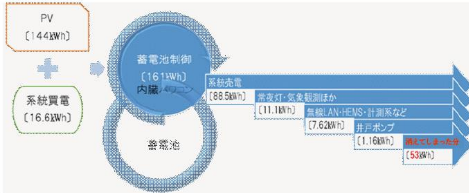
羽根木テラスBIOのリチウムイオン電池のパフォーマンス（注）測定（2015年8月から2016年7月）とその結果の解析は(株)環境エネルギー総合研究所による
