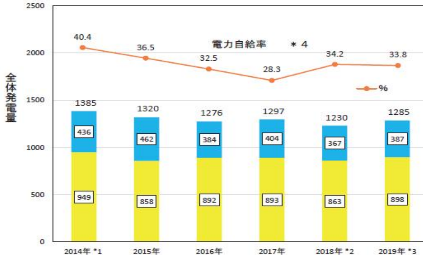
羽根木エコハウスの直近6年間の太陽光発電とその用途内訳の推移(単位：kWh、%)
